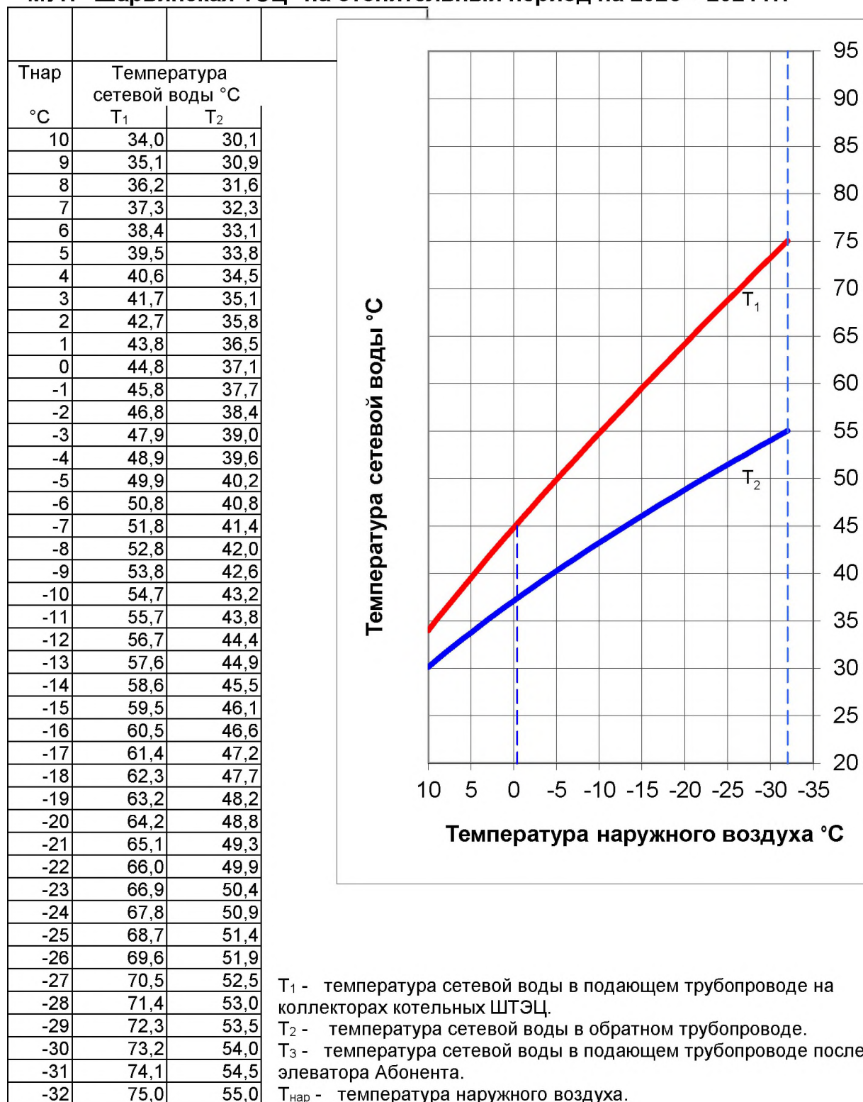
Рисунок 5.5.2 – Температурный график тепловых сетей от муниципальных котельных.
